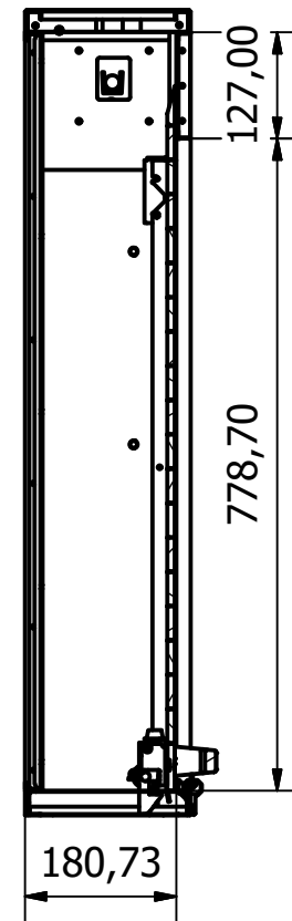
C-C ( 1 : 10 )
