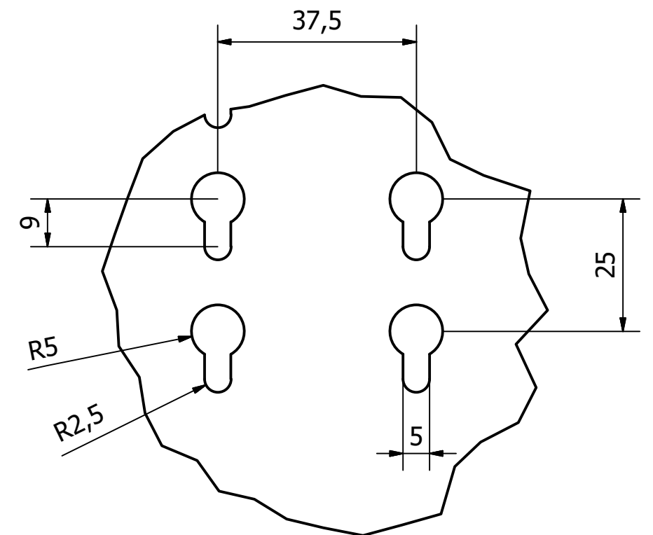
A ( 1 : 1 )
